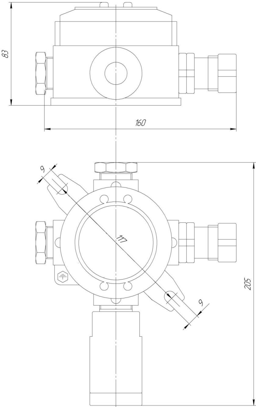
Рисунок 1. Габаритный чертеж прибора
